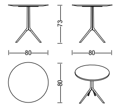
FR80A Tavolino tondo 80 cm H73 cm Round table 80 cm H73 cm
